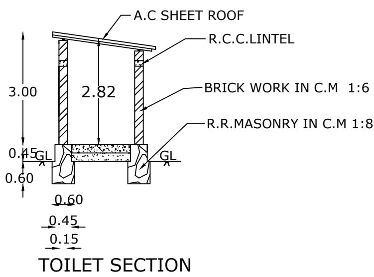
TOILET SECTION
