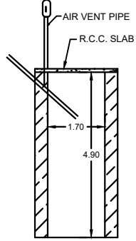
SOAK PIT
