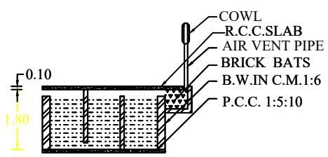
S.T SECTION
