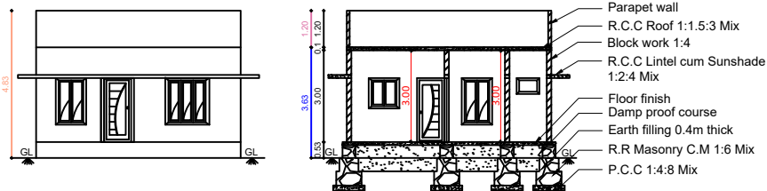
ELEVATION
