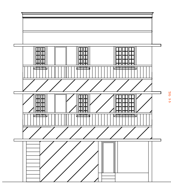
ELEVATION
