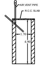
SOAK PIT
