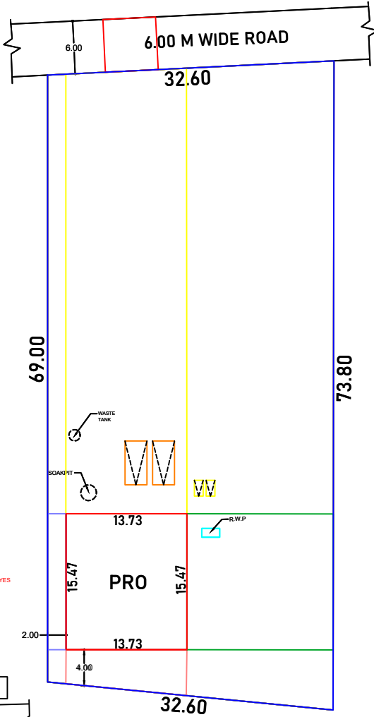
SITE PLAN (SCALE 1:250)
