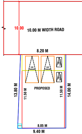
SITE PLAN SCALE 1:100
