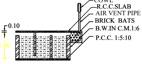
S.T SECTION
