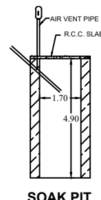
SOAK PIT
