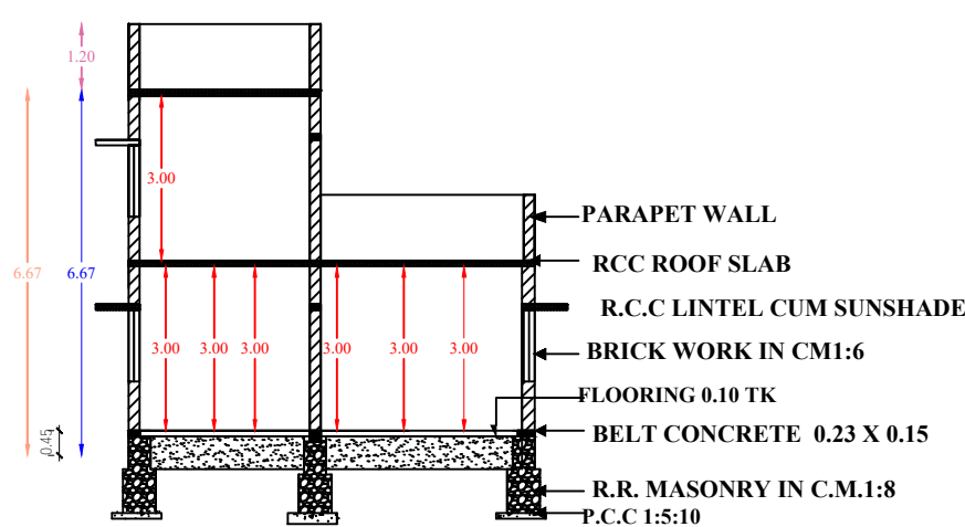
SECTION A-B
