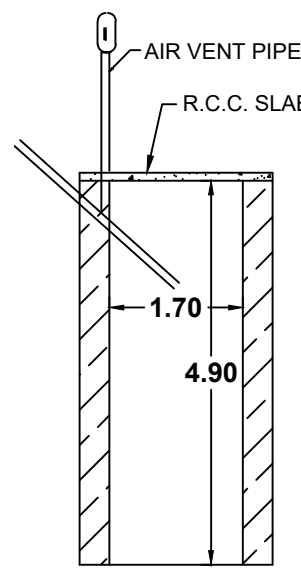
SOAK PIT
