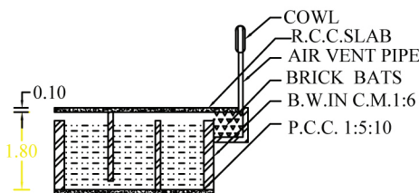
S.T. SECTION
