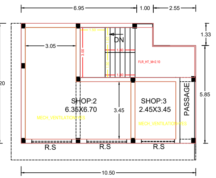
F.F.PLAN
