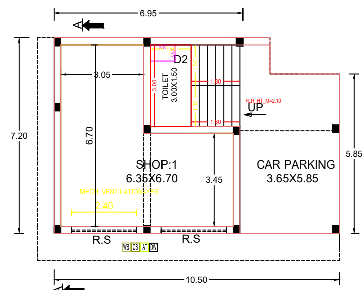
G.F.PLAN
