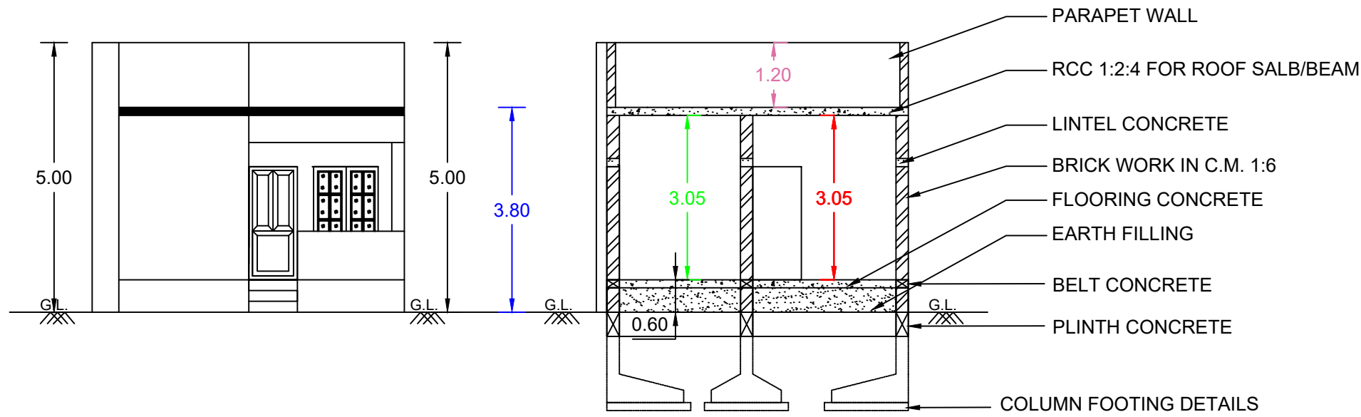
ELEVATION
