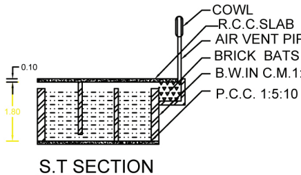
S.T. SECTION
