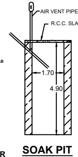
SOAK PIT
