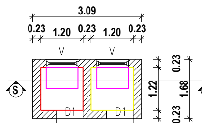
TOILET PLAN
