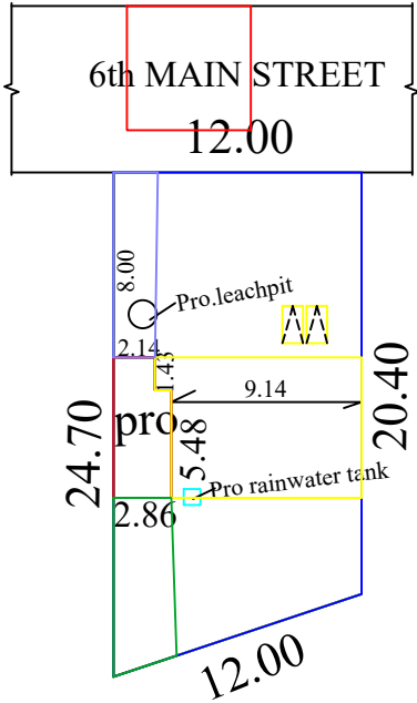
SITEPLAN SCALE : 1:200
