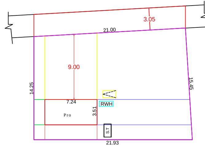
SCALE 1:100 SITE PLAN
