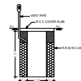
SOAK PIT
