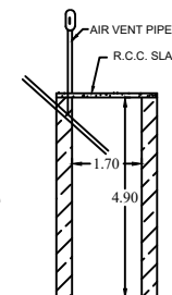
SOAK PIT
