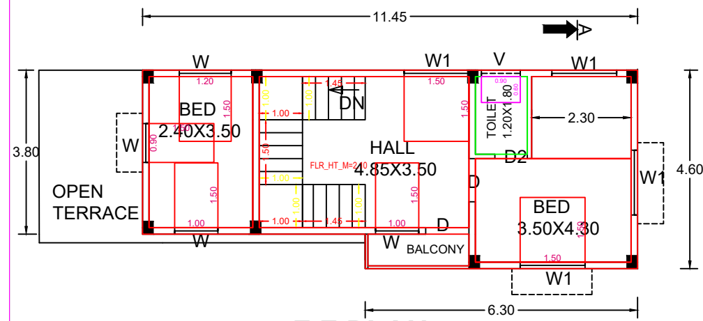
F.F. PLAN
