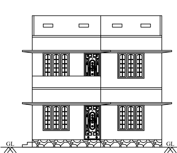
ELEVATION
