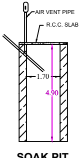
SOAK PIT
