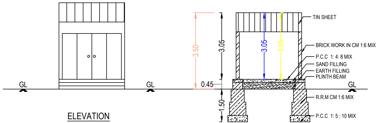
ELEVATION
