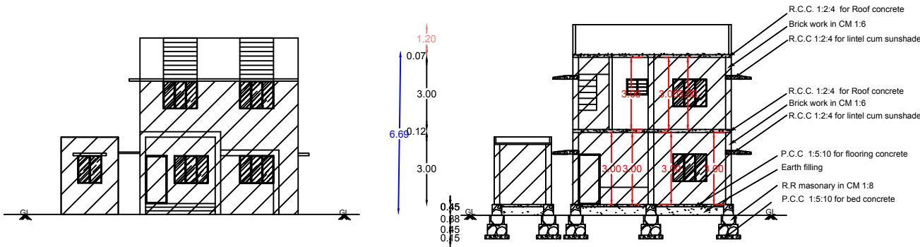
ELEVATION
