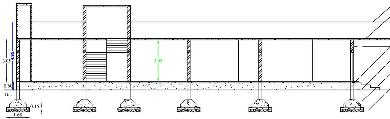
SECTION 'AB'
