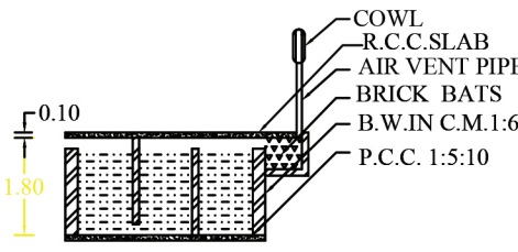
S.T. SECTION
