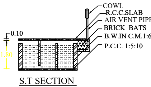
S.T. SECTION
