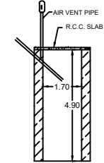
SOAK PIT
