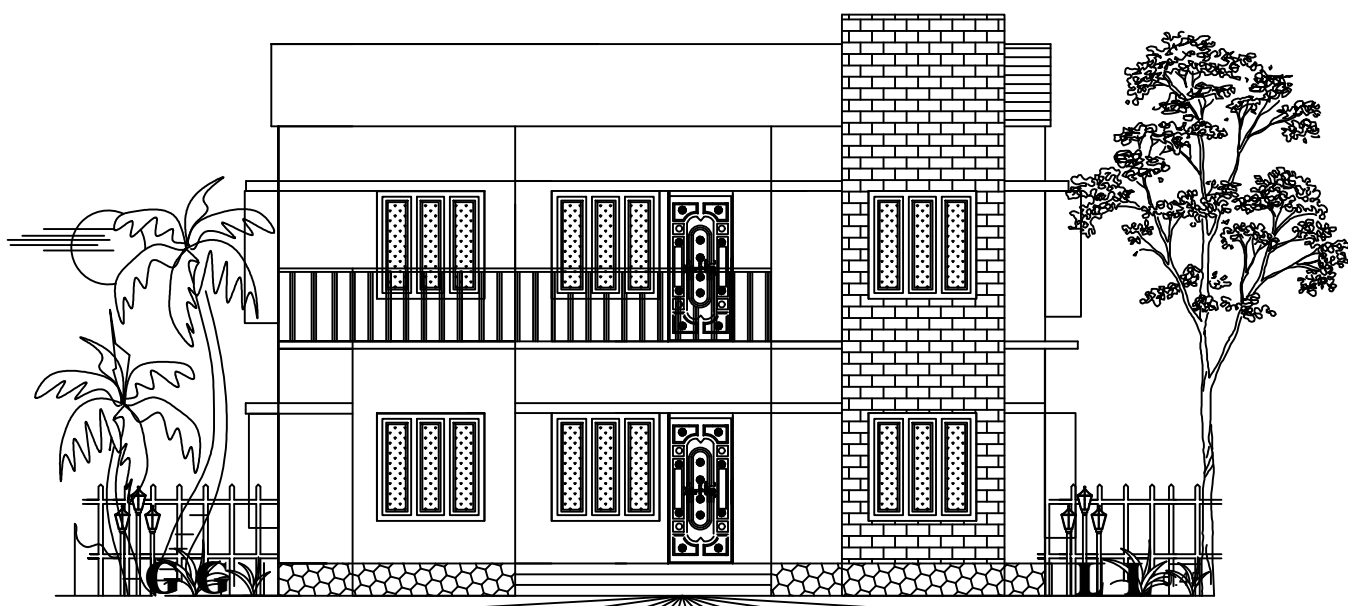
ELEVATION
