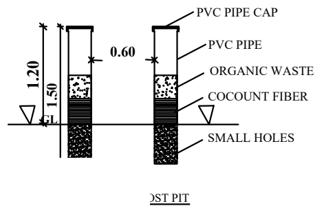
SOAK PIT
