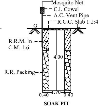
SOAK PIT
