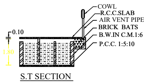
S.T. SECTION
