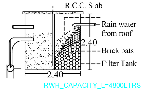
RWH_CAPACITY_L=4800LTRS
