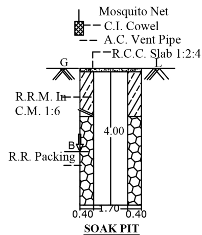
SOAK PIT
