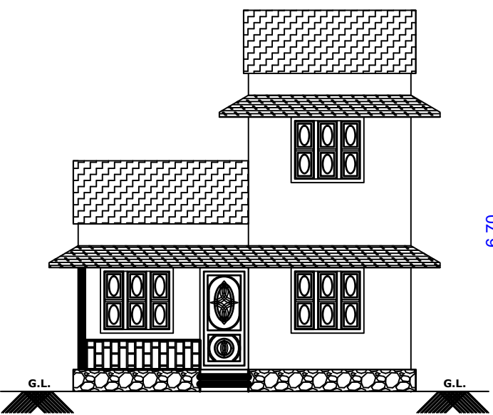
ELEVATION
