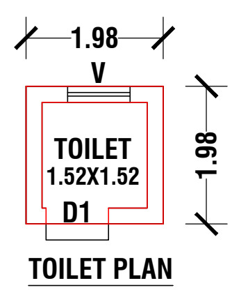
TOILET PLAN
