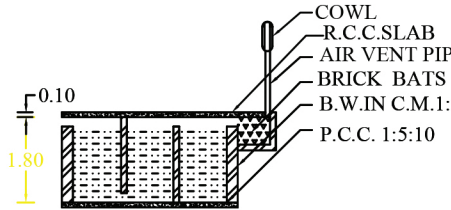
S.T SECTION
