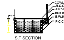
S.T. SECTION
