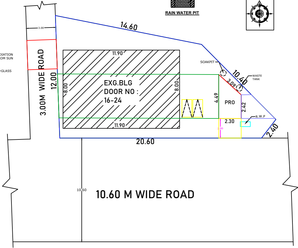
SITE PLAN(SCALE 1:100)
