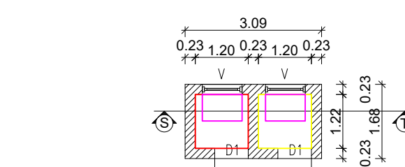
TOILET PLAN
