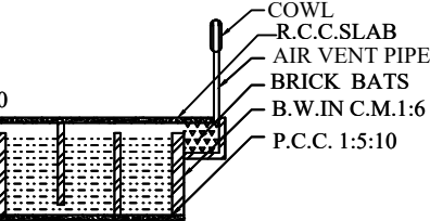
S.T SECTION
