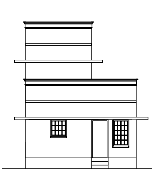
ELEVATION
