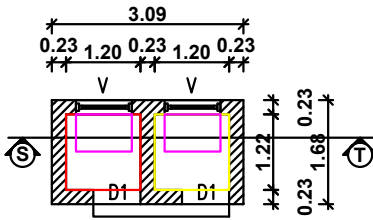
TOILET PLAN
