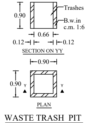
SECTION ON Y Y
