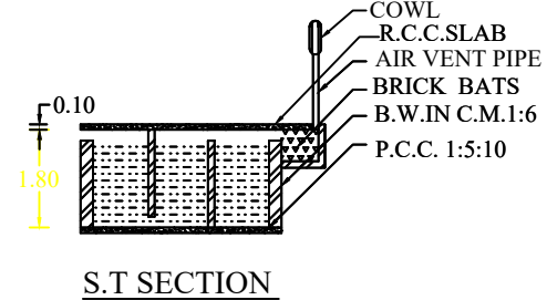
S.T SECTION
