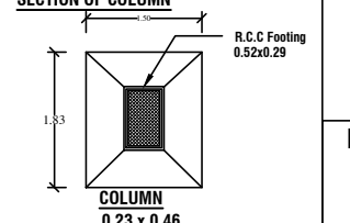
COLUMN 0.23 x 0.46
