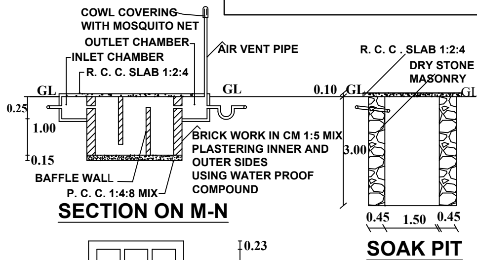
SOAK PIT
