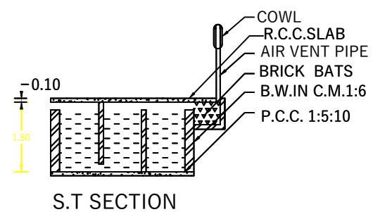
S.T SECTION
