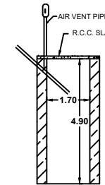
SOAK PIT
