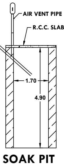
SOAK PIT
